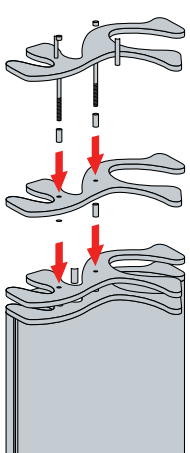
Befestigung eines Endplatten-Erweiterungs-Sets an die Organic-Stütze
